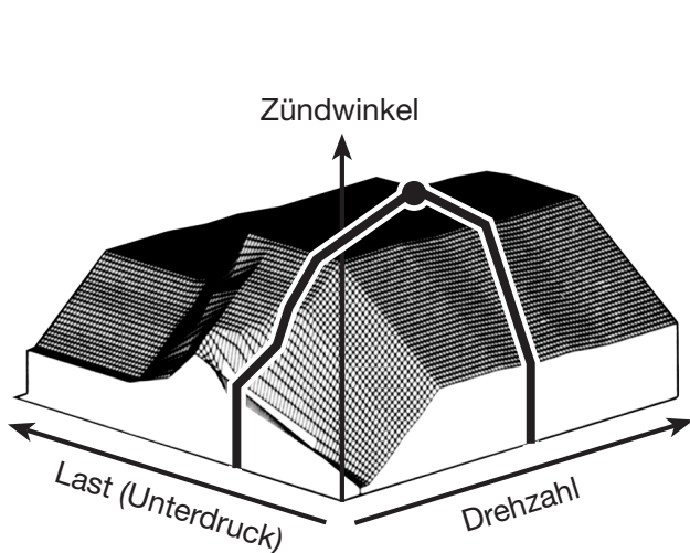
Zündkennfeld eines mechanischen Verstellsystems:
